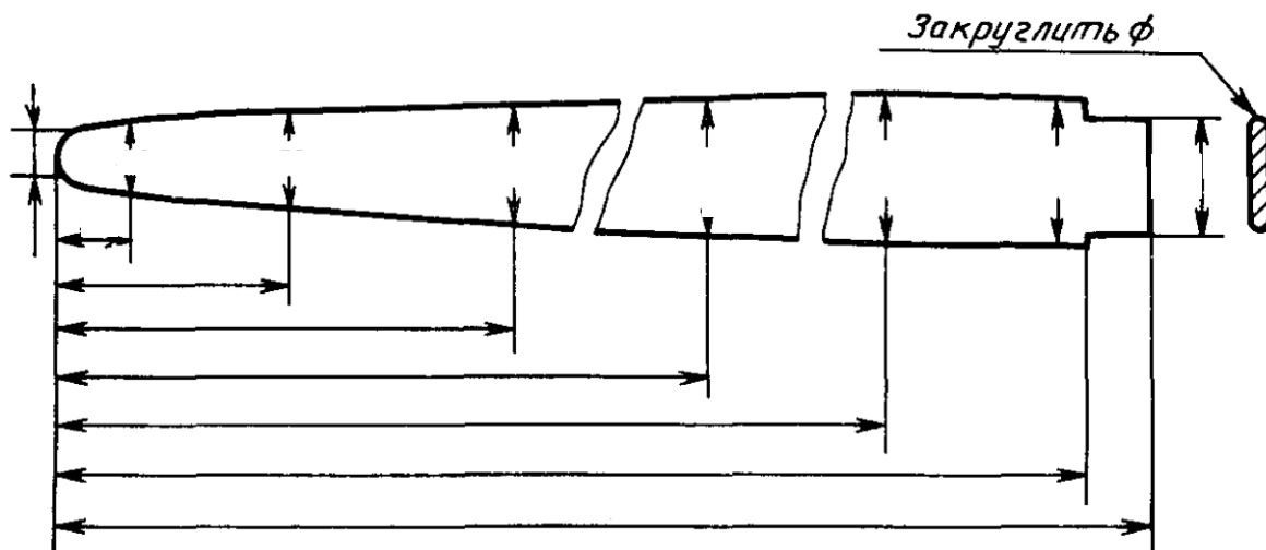
Рисунок Б.1 – Правилка для шкурок норки
